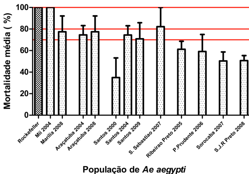
Gráfico 3. Percentual médio de mortalidade de populações de Aedes aegypti expostas ao tratamento com larvicida temephos, segundo origem e ano de avaliação.
