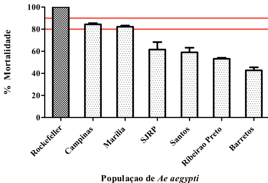
Gráfico 4. Percentual médio de mortalidade observado em populações de Aedes aegypti expostas em gaiolas sentinelas ao tratamento com cipermetrina (dose 0,6 g i.a/imóvel). Provas realizadas em 2000/2001.
