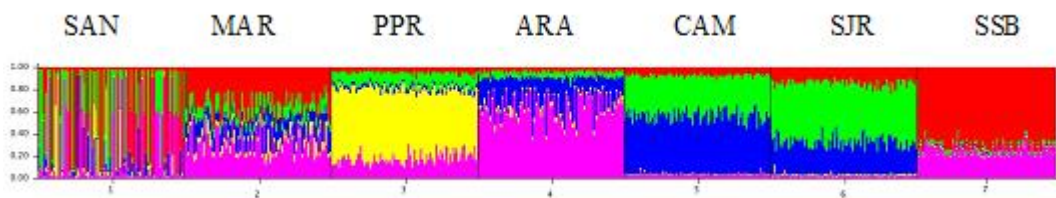
Figura 1. Análise genética de sete populações sentinelas do Estado de São Paulo.
