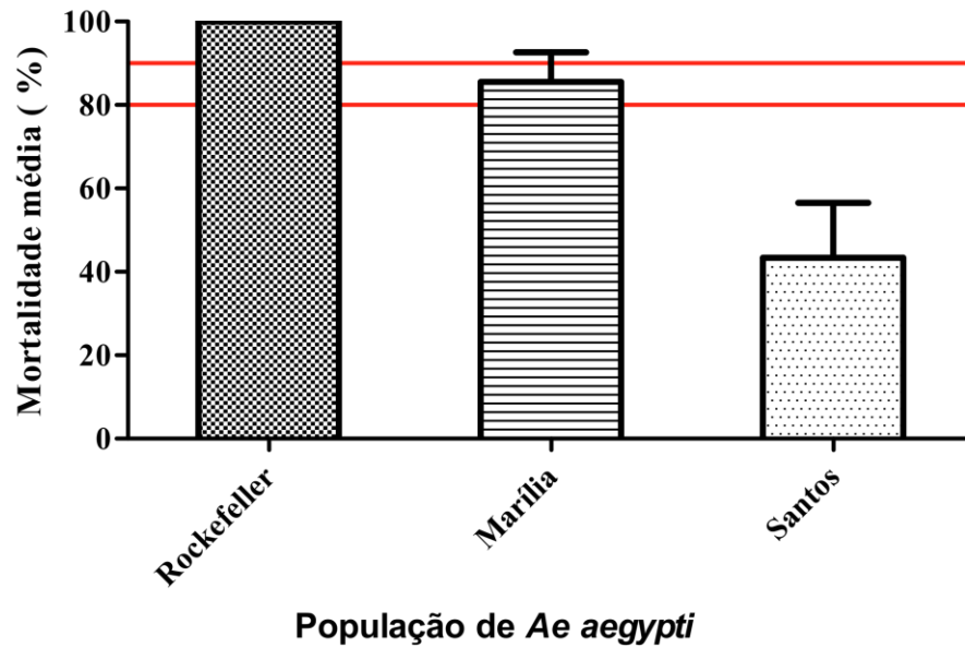
Gráfico 5. Percentual médio de mortalidade em populações de Aedes aegypti em tratamento espacial com permetrina. Provas realizadas em 2002.
